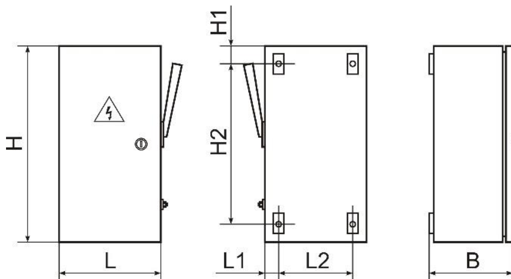
Общий вид и габаритные размеры ящиков силовых серии ЯВЗ.
